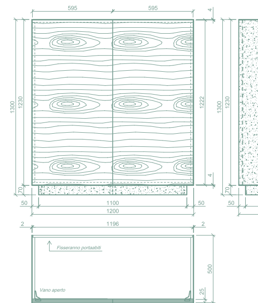
SEZ. ORIZZONTALE
